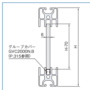
スライドアパネル加工寸法
