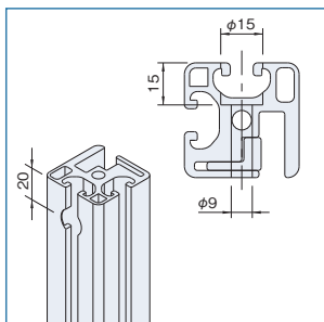
接続する相手側は、φ15ザグリ深サ15mm φ9トオン(加工品番 CP15)の加工をしてください。
