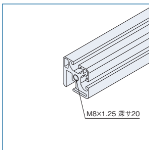
ジョイントの取付側は、M8x1.25 深サ20mm(加工品番 M8x20)のタップ穴加工をしてください。
