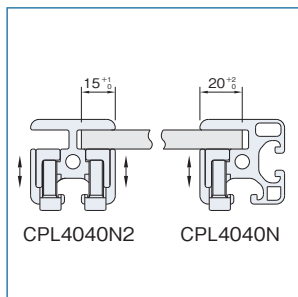
パネルエレメントの適した差し込み深さ。
