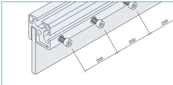
200mmピッチでザグリタップ穴加工済み。
