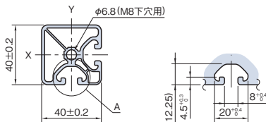
詳細 A
