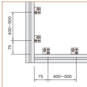
マルチブロックの取付方法。
