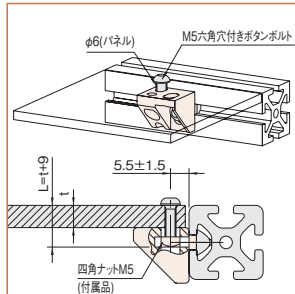
パネルの取付方法1 (M5ボルト使用)。
