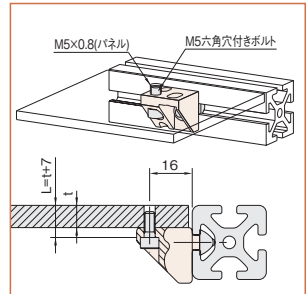
パネルの取付方法2 (M5ボルト使用)。
