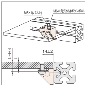
パネルの取付方法3 (M6ボルト使用)。
