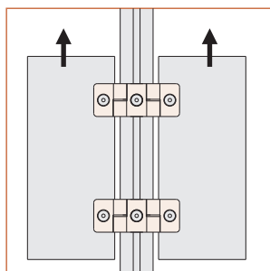
両開き(L6-DHL7830使用)
