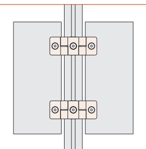
左開き(L6-HLD4830L使用)
