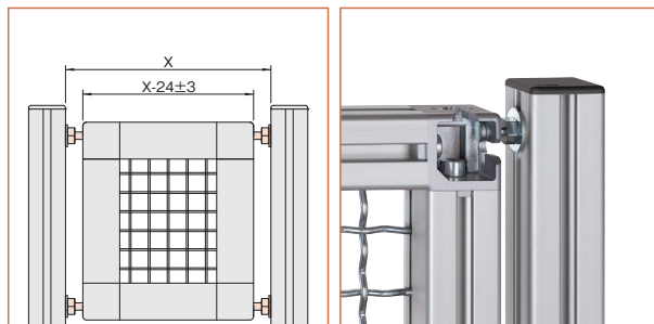
パネルユニット取付け例。
