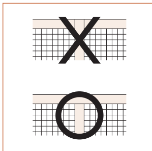
間仕切りでは、上図の様に突き出さないでください。縦方向の間仕切り
