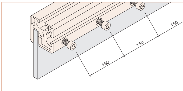
150mmピッチでザグリタップ穴加工済み。
