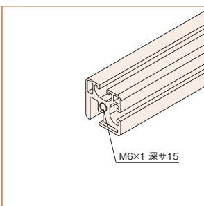
ジョイントの取付側は、M6×1 深サ15mm (加工品番 M6×15)のタップ穴加工をしてください。
