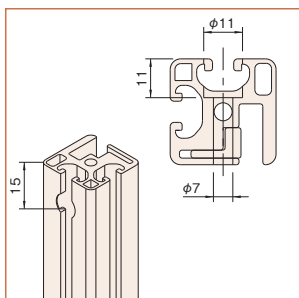
接続する相手側はφ11ザグリ深サ11mmφ7トオリ加工品番 CP11)の加工をしてください。
