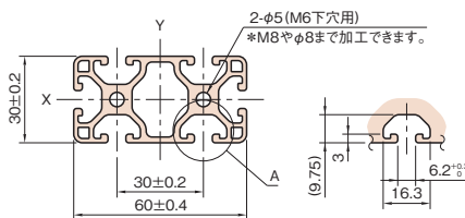
詳細 A
