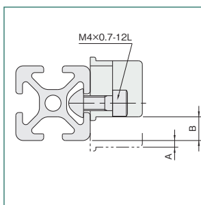
L5-SPH2020Nに取付けた場合の取付位置 A=1mm、B=7mm。
