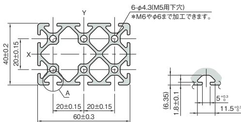
詳細 A
