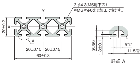
詳細 A
