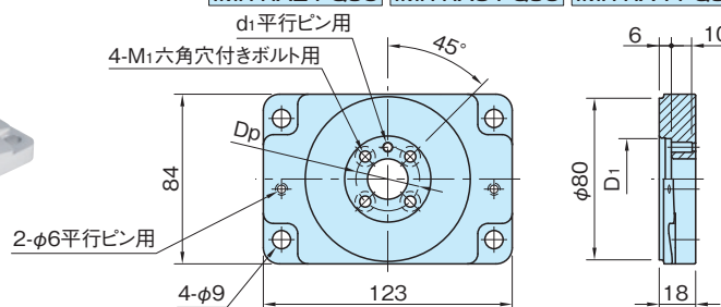
IMR-RA4-PQ9020
