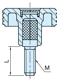
GK-N (オネジ)
