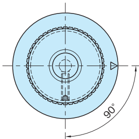
GCKFP (矢印フランジ付き)
