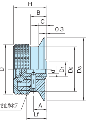
GCKFM (目盛りフランジ付き)
