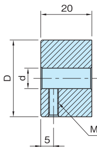
ESR1R (目盛り方向:右)
