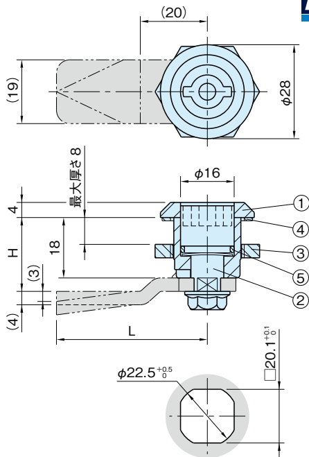
取付穴図
