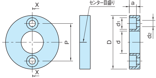
断面 X-X
