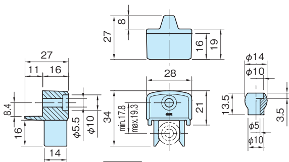
DLB30 (本体・ボール)
