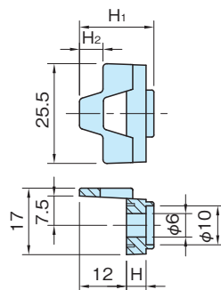
DLB30-05~15 (スペーサー)
