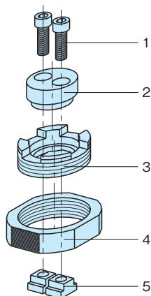
部品構成
