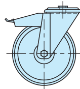
CAG1-FBF (旋回,通し穴,ストッパー付き)
