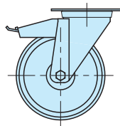
CAG1-SBF (旋回,プレート,ストッパー付き)
