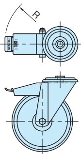
CAFF-FBF CAFF-FBF-SUS (旋回,通し穴,ストッパー付き)
