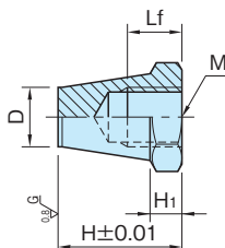
BJ810-F (先端研磨タイプ)
