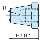
BJ810-R (先端Rタイプ)
