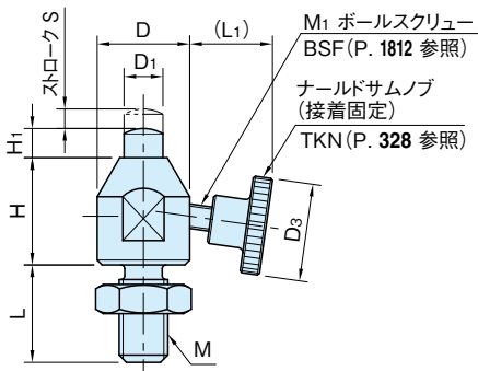
BJ360**001 (ナールドサムノブ仕様)
