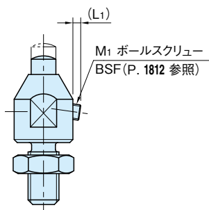
BJ360**002 (ボールスクリュー仕様)
