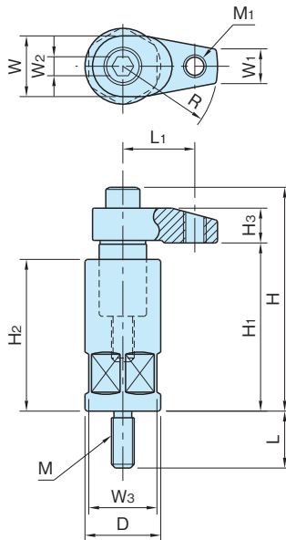
M12タイプ
