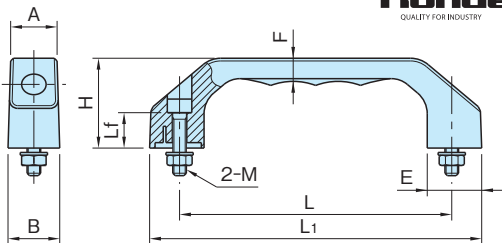
AG1 (六角穴付きボルト仕様)
